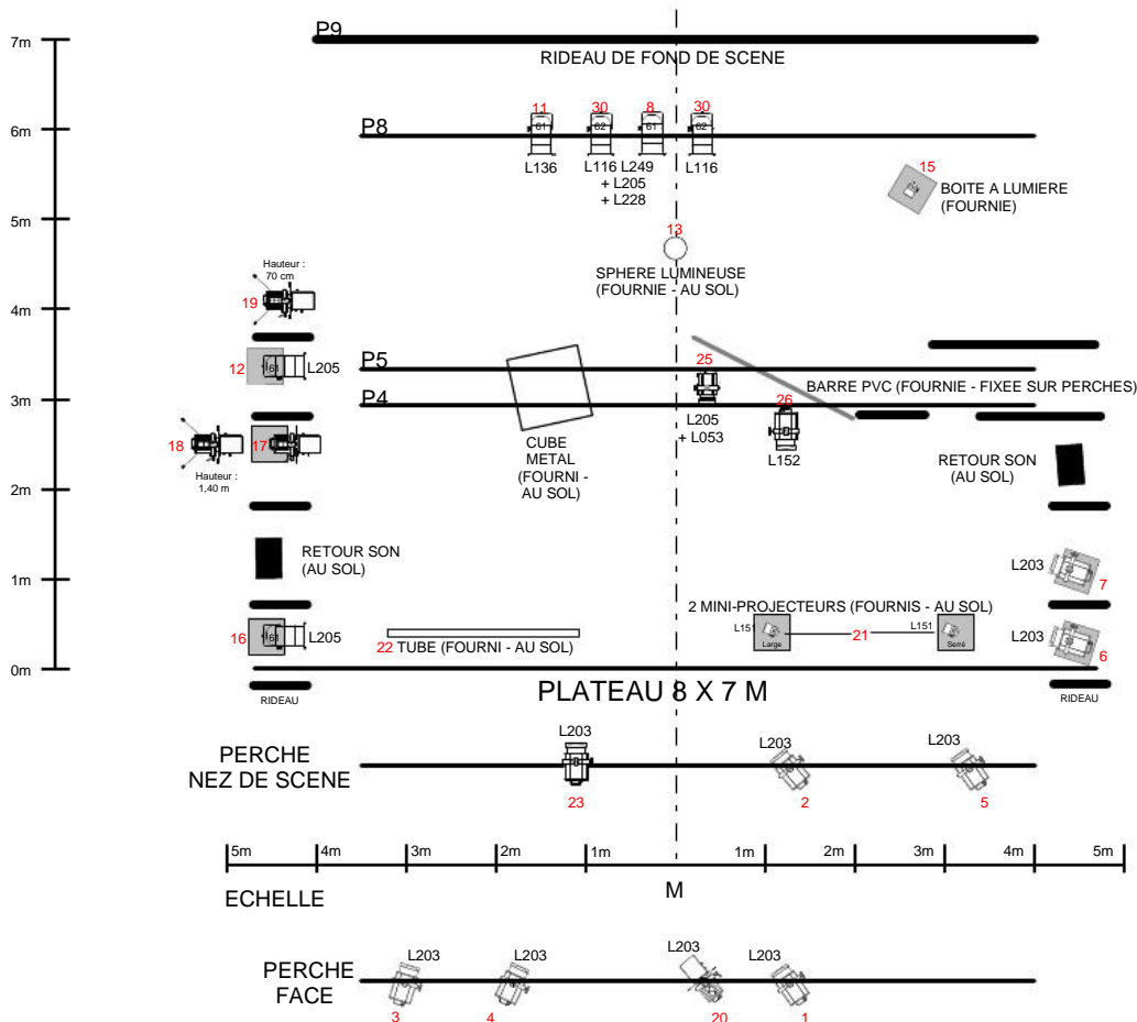
COMPAGNIE MOI NON PLUS "LE BAL DES GRENOUILLES" PLAN DE SCENE
